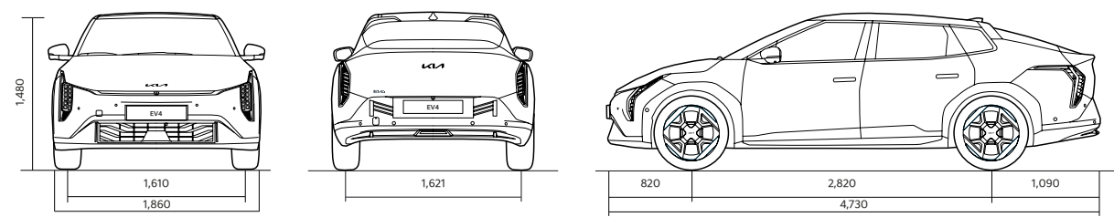
Afmetingen Fastback
