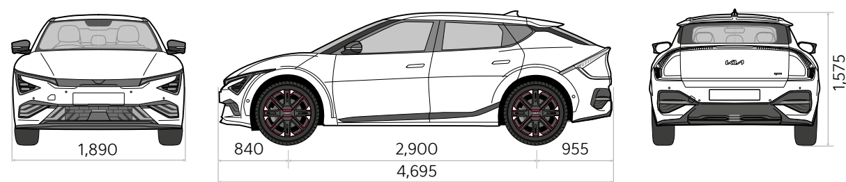
Afmetingen GT-Line
