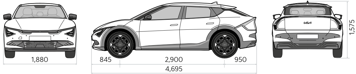
Afmetingen GT-Line
